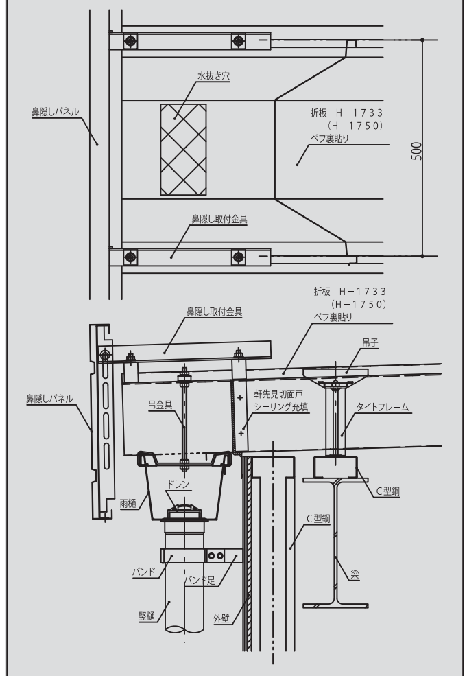
■軒先部納まり（鼻隠し）
