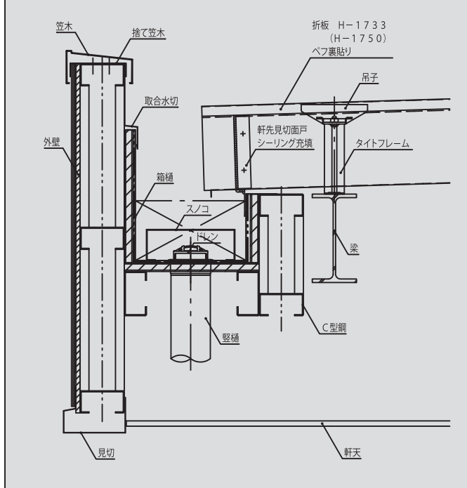
■軒先部納まり
