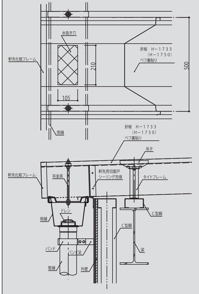
■軒先部納まり
