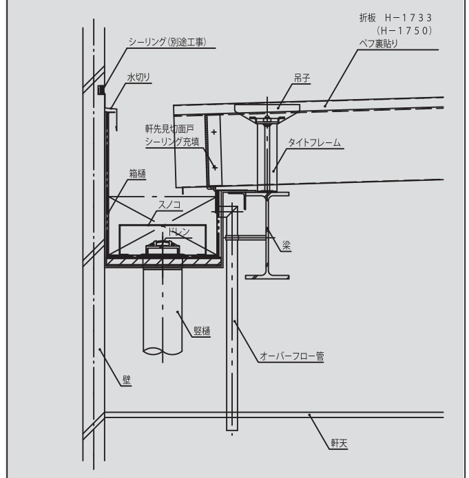
■軒先部納まり
